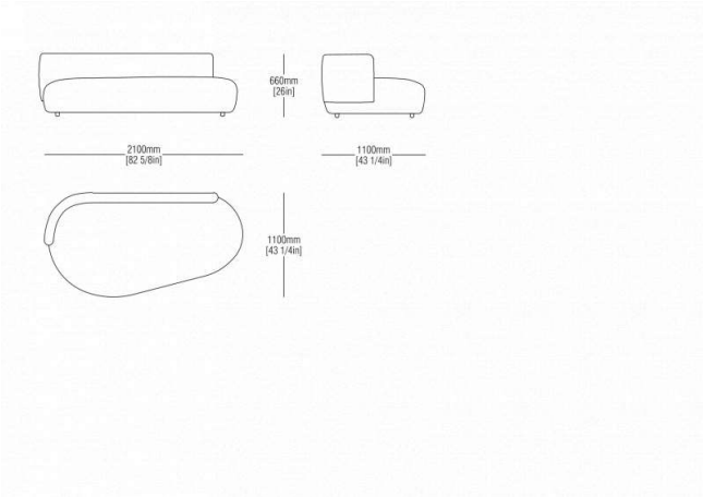
Sofa W. 2100 mm
