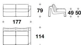
ING (E2D) - ING (E2S) ELEMENTO 2 POSTI CON BRACCIOLO DX O SX / 2 SEATER ELEMENT WITH RIGHT OR LEFT ARMREST 177x114x79H. - H.A.50 - H.S.49cm 69 2/3x45x31H. - H.A.19 3/4 - H.S.19 1/4"
