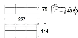
ING (E3D) - ING (E3S) ELEMENTO 3 POSTI CON BRACCIOLO DX O SX / 3 SEATER ELEMENT WITH RIGHT OR LEFT ARMREST 257x114x79H. - H.A.50 - H.S.49cm 101 1/3x45x31H. - H.A.19 3/4 - H.S.19 1/4"
