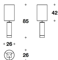
DMP (10) HIGH : LAMPADA DA TAVOLO CON BASE QUADRATA / TABLE LAMP WITH SQUARE BASE Ø 26x85H. cm Ø 10 1/4x33 1/3H. "
